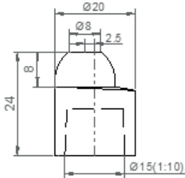
2000 412 810 exzentrisch
