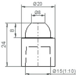
2000 412 809 zentrisch
