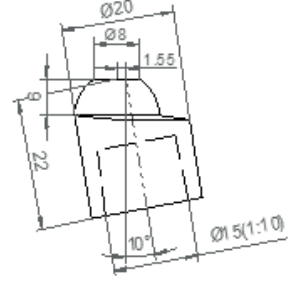
2000 120 929 exzentrisch 10°
