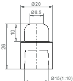
R100 149 380 zentrisch
