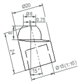
2000 412 812 exzentrisch 15°
