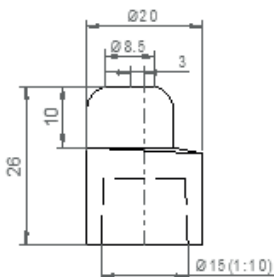
R100 149 382 exzentrisch
