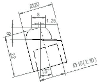
P911 321 205 exzentrisch 15°
