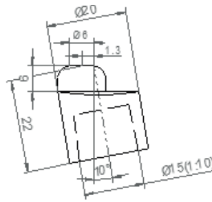
2000 358 777 exzentrisch 10°
