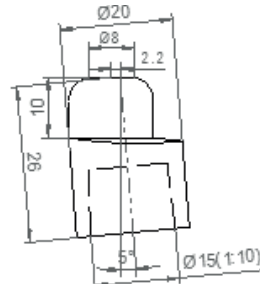
R100 149 383 exzentrisch 5°
