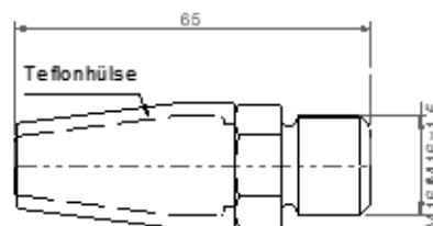
S-3941 mit Teflonisolierung
